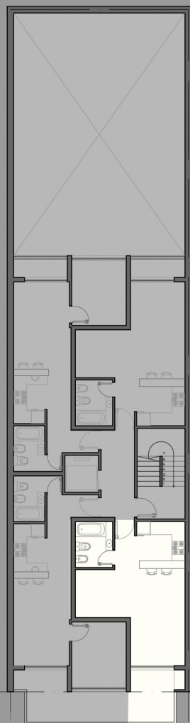
PLANTA TIPO
