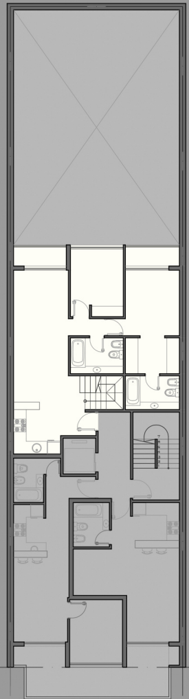
PLANTA 6° PISO
